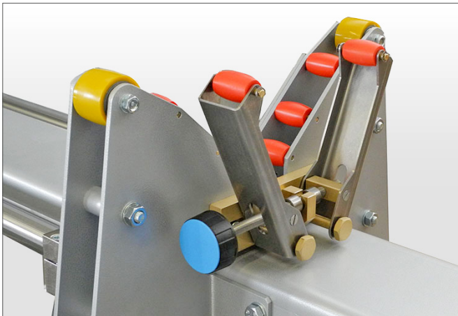
Gestell mit einer V-förmigen Auflage
